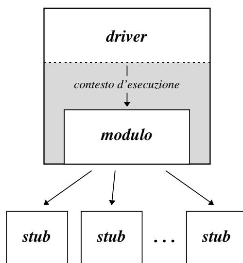
Fig. 2.3. Driver e stub nel test di un modulo.
