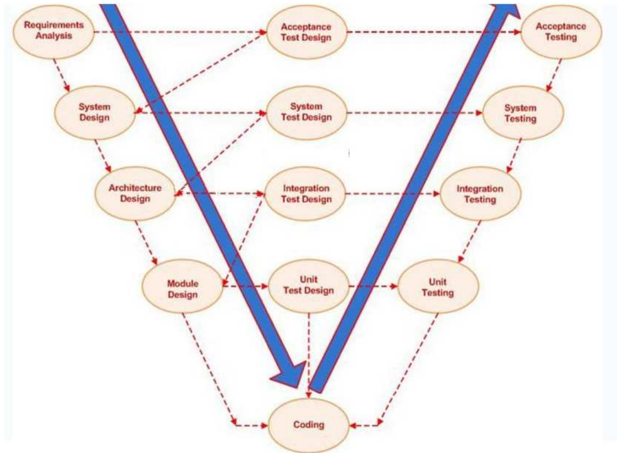
Fig. 2.5. Il V-Modell. (cortesia di Wikipedia)
